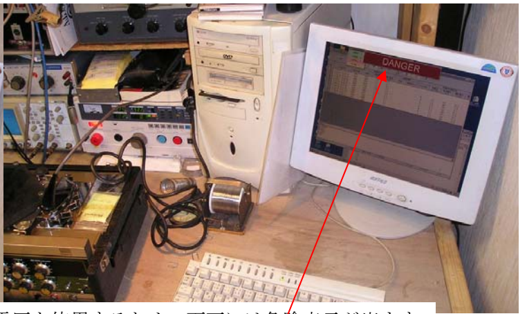
電気試験準備完了と試験開始 1000vもの高電圧を使用するため、画面には危険表示が出ます
